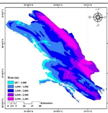
شکل ۴. لایه ارتفاع
