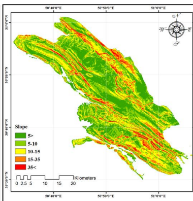
شکل ۷. لایه شیب
