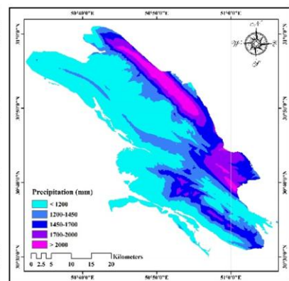
شکل ۳. لایه بارش
